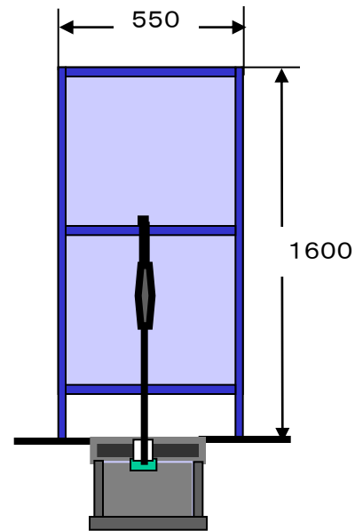
標準立看板設置図
